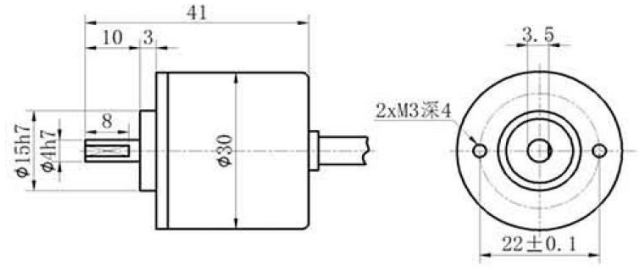
尺寸单位为毫米，若无特殊说明，尺寸公差为±0.5mm Dimensions in mm. Unless otherwise stated, tolerance: ±0.5mm
